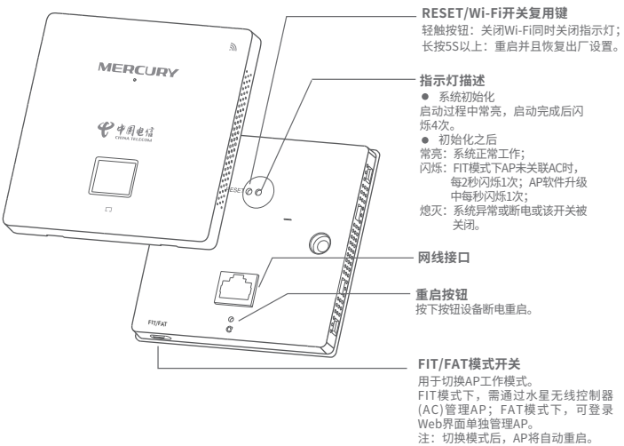
正面示意图
